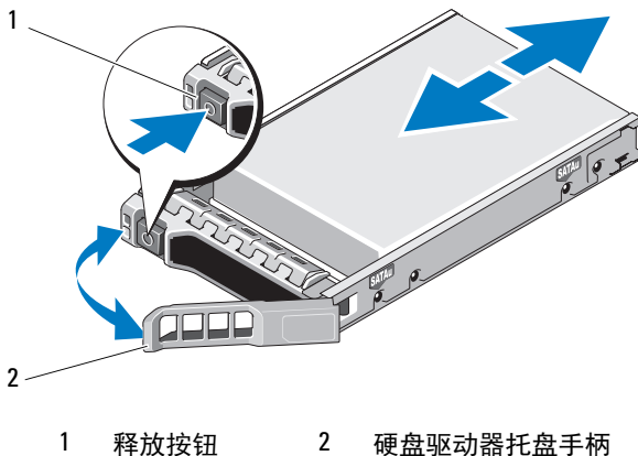
图 16-4. 卸下和安装硬盘驱动器
